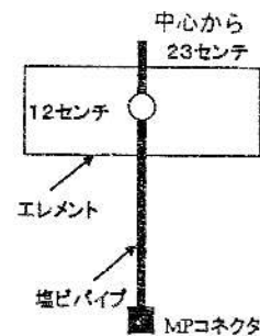
2/3λ 430MHz ヘンテナ 試作: JA7CWI
